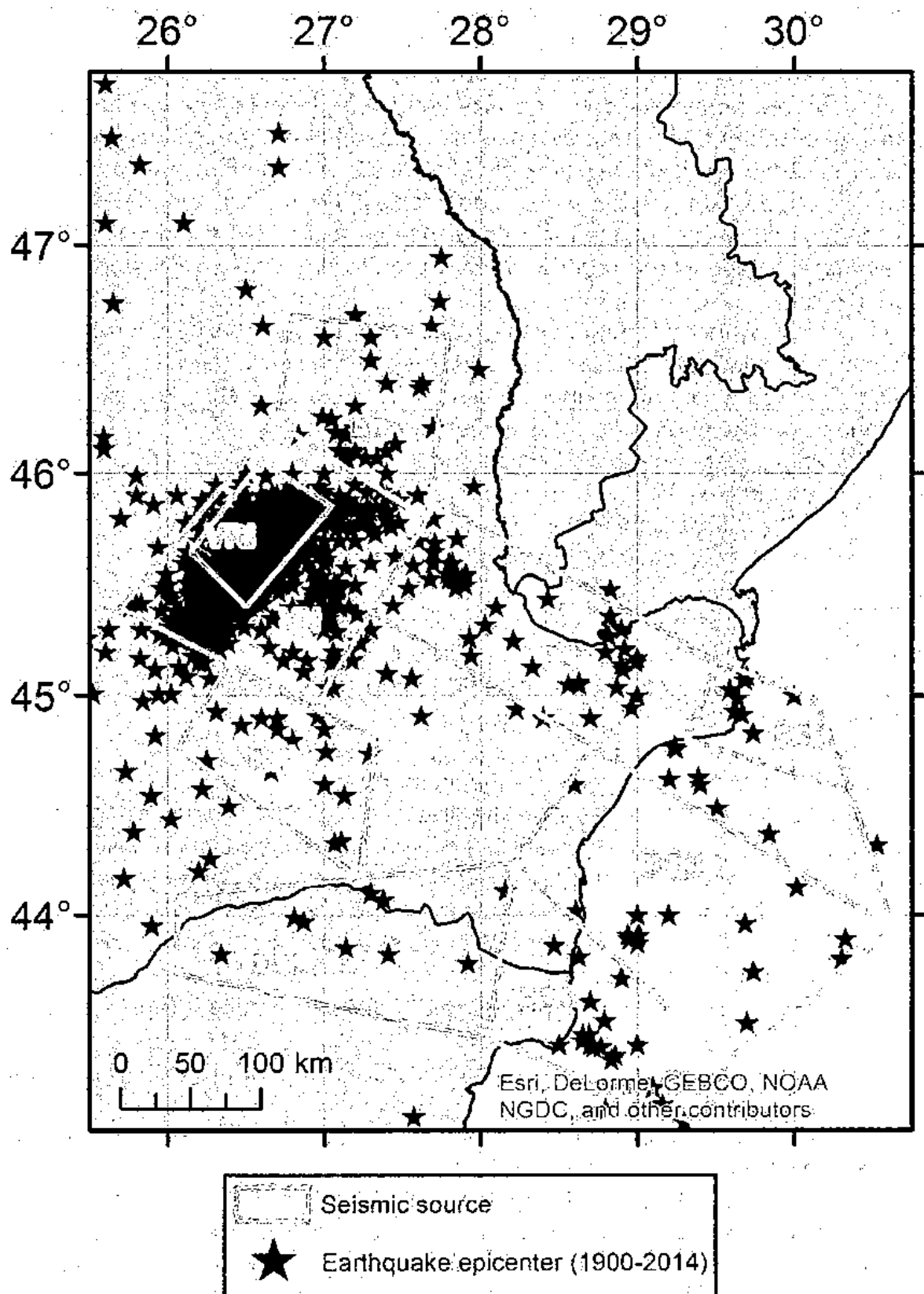
Figura 2. Detaliu cu sursele seismice marine din apropierea litoralului românesc al Mării Negre. Au fost folosite doar cutremurele cu M_w > 3.5 pentru sursele de pe uscat,
