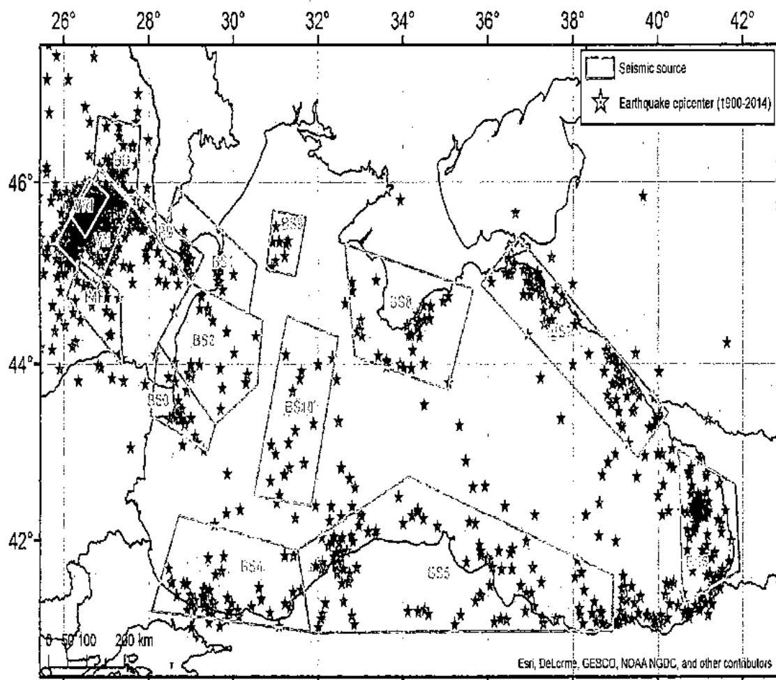
Figura 1. Zonarea seismică pentru partea de E a României și pentru zona Mării Negre
