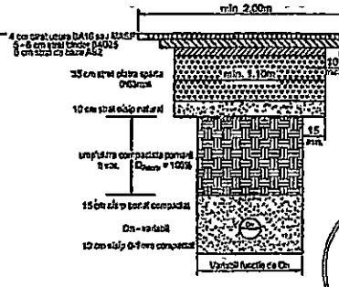
SECTIUNE TIP T2 STRAZI CU TRAFIC GREU
