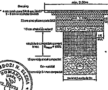
SECTIUNE TIP T3 STRAZI CU TRAFIC MEDIU
