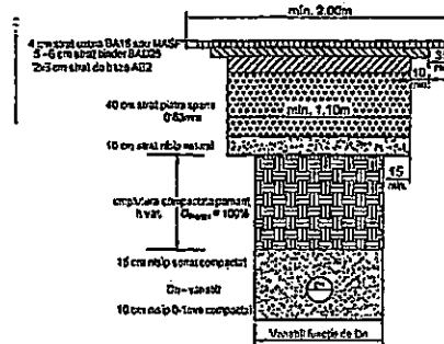
SECTIUNE TIP T1 STRAZI CU TRAFIC FOARTE GREU
