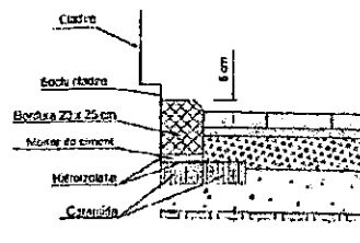
Detaliul "A"
