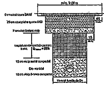
SECTIUNE TIP T5 STRAZI CU TRAFIC FOARTE USOR
