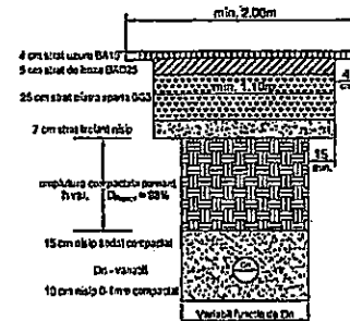
SECTIUNE TIP T4 STRAZI CU TRAFIC USOR
