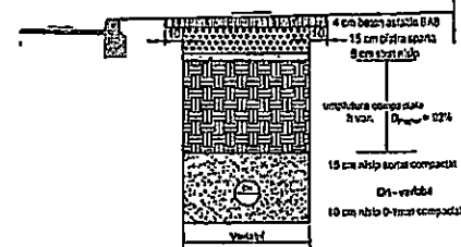
REFACERE ÎMBRĂCĂMINTE TROTUARE
