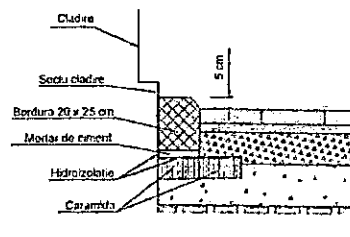
Detaliu "A"
