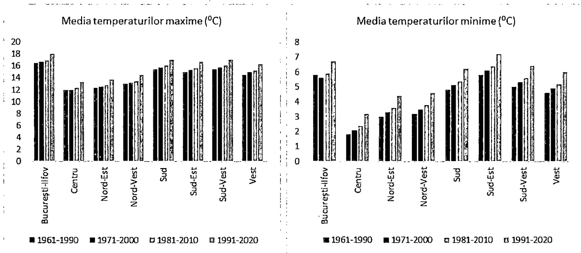
Figura 71: Schimbări în mediile temperaturii maxime (stânga) și minime (dreapta) anuale în diferite perioade de referință de 30 ani în regiunile de dezvoltare ale României
