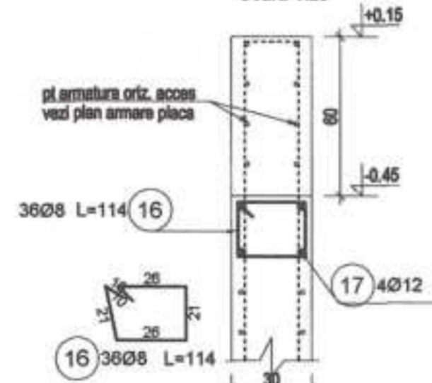
Centura pereti in zona acces Scara 1:20
