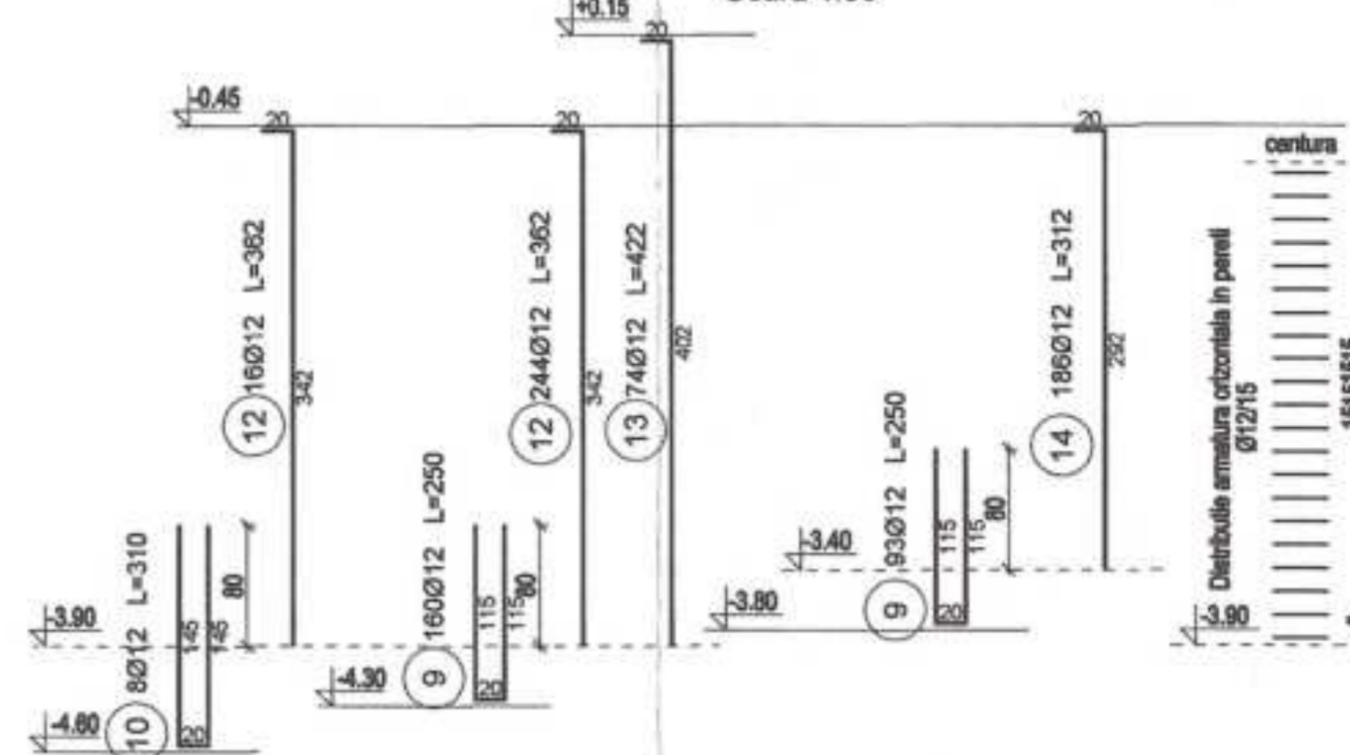
Fila bare Scara 1:50
