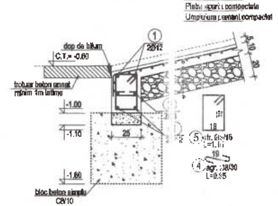
Secțiunea 2-2 sc. 1:20
