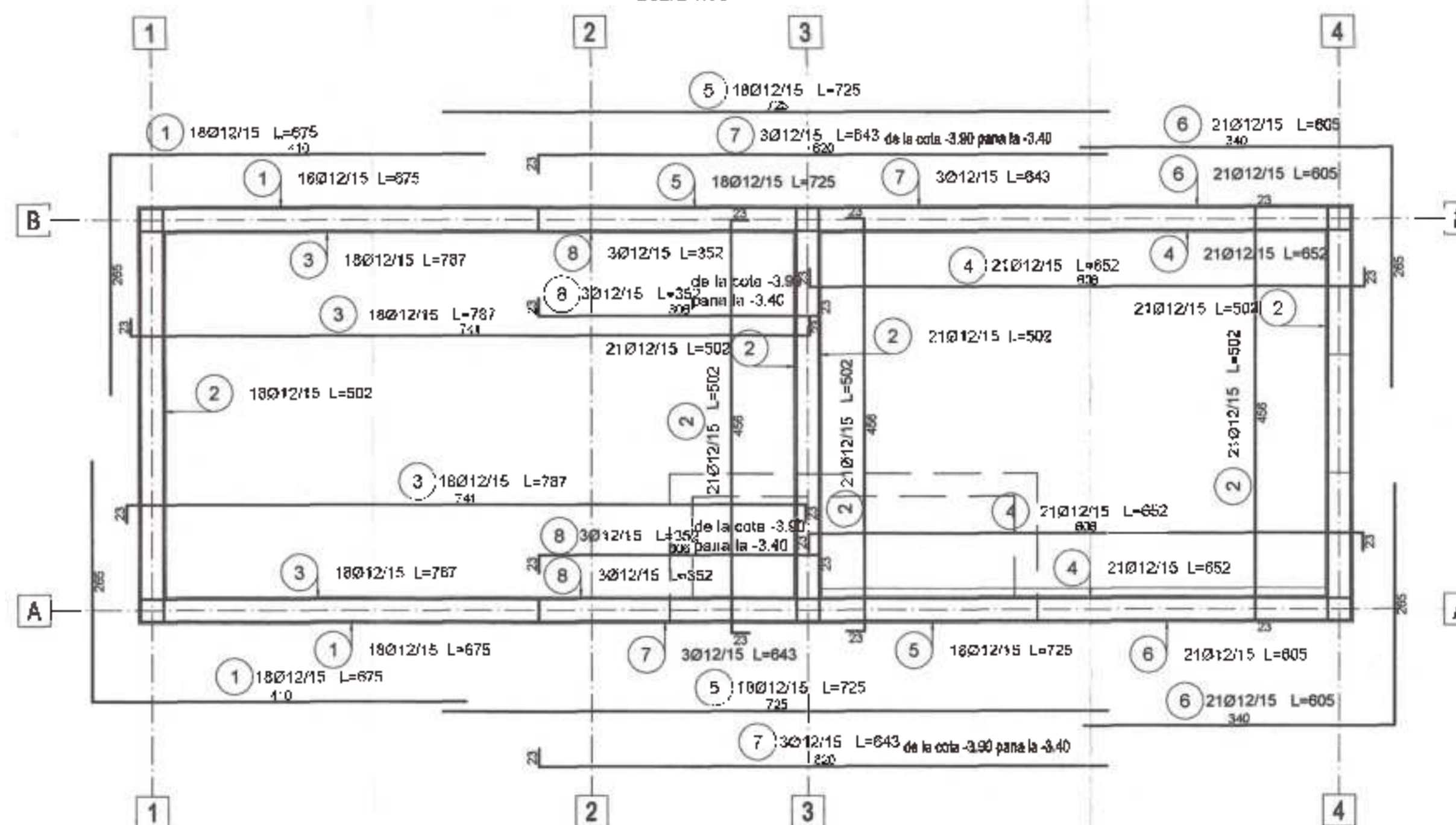
Plan armare orizontala pereti Scara 1:50
