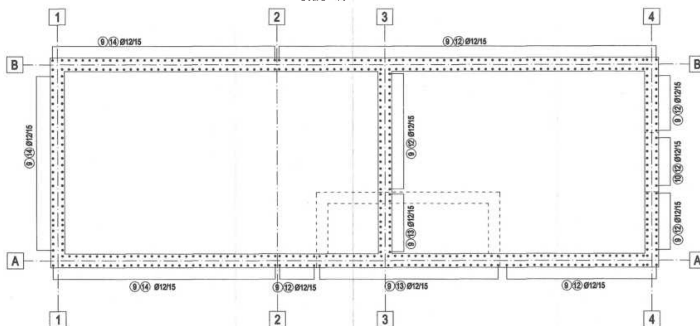
Plan armare verticala pereti Scara 1:50
