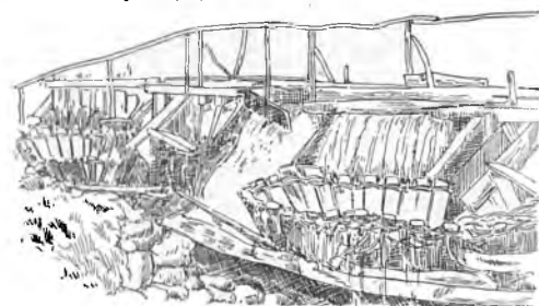
Fig. 5315. Viltoare (după Tache Papahagi).
