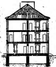
Fig. 4401. Secțiunea unei clădiri.
