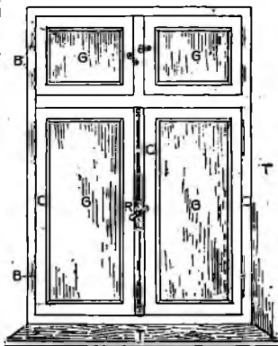
Fig. 2071. Fereastră. C. C. Cercevele.—G. G. Geamuri. — T. T. Toc, pervaz. — R. Cremonă. — B. B. Țigini.
