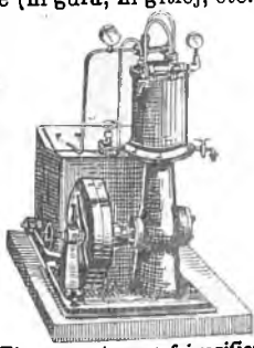
Fig. 2211. Aparat frigorific
