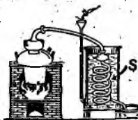
Fig. 4424. S. Serpentin.
