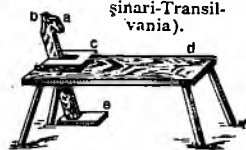
Fig. 4337. Scaun de doage. (ab. clește; -c. măsujă, pod, punte; -d. scaun; -e. calcător, tălpigă).
