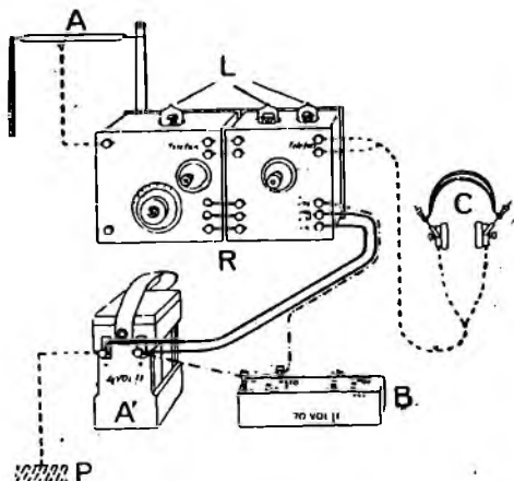
Fig. 4066. Instalațiunea unui post receptor de radiofonie. A. Antenă. — P. Legătura antenei cu pămîntul. — A'. Acumulator. — B. Baterie anodică. — R. Aparat de recepție L. Lămpi. — C. Cască.
