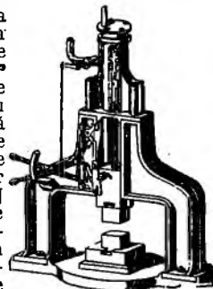
Fig. 1188. Cioacan cu aburi.
