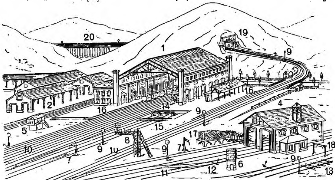
Fig. 2303. Gara. 1. Gara. — 2. Gara de mărfuri. — 3. Marchiză. — 4. Remiză pentru locomotive. — 5. Post de acar. — 6. Rezervor. — 7. Friză de apă. — 8. Semafor. — 9. Disc. — 10. Şine. — 11. 12. Macazuri. — 13. Traverse. — 14. Parapet. — 15. Plăci turnante. — 16. Peron. — 17. Peronul cărbunilor. — 18. Gabarit. — 19. Tunel. — 20. Viaduct.
