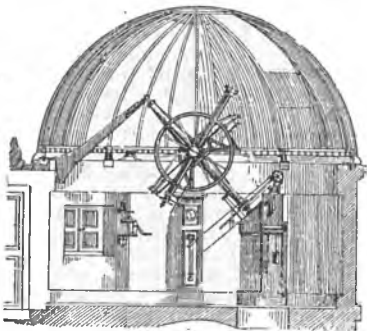
Fig. 1957. Ecuatorial.
