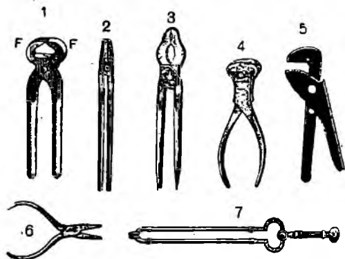
Fig. 1291. Clești: 1. Clește de timplă, de dulgher (F. F. fălei). — 2. 3. Cl. de fierar, de lăcătuș. — 3. Cl. de mecanic. 4. Cl. de cizmar. — 5. Cl. pentru sîrmă. — 6. Cl. de soba. — 7. Cl. de soba.
