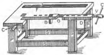
Fig. 4861. Tejghea de timplar. F. Față, blană, masă. — J. Jghiabul uneltelor, șant, gavan, uluc. — P.P. Picioare. — S.S. Stinghii, chingi. — V.V. Virtejuri, clești, șurupuri. — C. Cuiul șurupului. — B. Bancașan. — G. Gura tejghelei. — D. Drug, broască, giscă.
