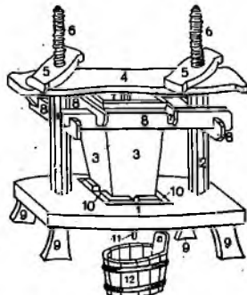
Fig. 4854. Teasc de struguri, 1. Masă, strat. — 2. Stîlpi. — 3. Coș, ladă, cutie. — 4. Grindă, punte. — 5. Giște, broaște. — 6. Șurupuri. — 7. Pop. — 8. Chingi, minii, argea, clește. — 9. Picioare. — 10. R. Jghiab, șant, vatră, girliciu. — 11. Țiță, burliu, uluc. — 12. Dejă, curătoare.
