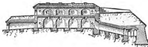
Fig. 1008. Interiorul unei cazemate.
