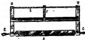
Fig. 2075, 2076. Ferestrae de dulgher. A. Dinți. — B. Pinză. — C. C. Miner. — D. Punte, chingă. — E. E. Brațe. — Pană, sucitor, cordar, etc. — S. Sfoară, coardă, strună. — U. U. Umeri, capete, cioace.
