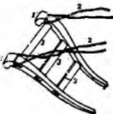
Fig. 1360. Codirlă. 1. 1. Cotoaie, cotoi, minuși. — 2. 2. Tînzători, lambe, lanțușuri, brăciri, baiere, curmeie, gujbe, ginjuri. — 3. 3. Spețeze.
