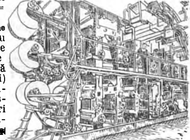
Fig. 4211. Mașină rotativă.
