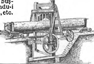
Fig. 2737. Joagăr.
