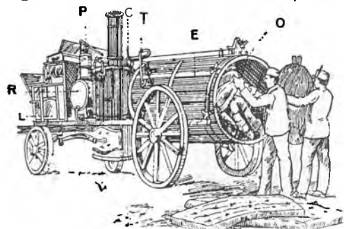
Fig. 2006. Etuvă. P. Pompă pentru desinfectarea locală. R. Rezervor de apă. L. Lada cu cărbuni. C. Cazan. T. Teava care duce aburii în etuvă. E. Etuvă. O. Obiecte de dezinfectat.
