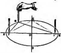
Fig. 1980. Construirea unei elipse.
