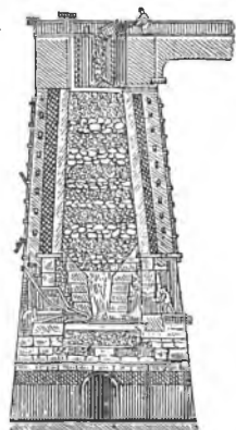
Fig. 1694. Cuptor înalt.
