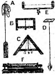
Fig. 1676. Cumpene. A. B. C. D. Cumpene verticale. — E. F. Cumpene orizontale.
