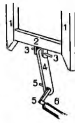
Fig. 2745. Jugul joagărului. 1.7. Vatale. — 2. Ceafă de jos. — 3.3. Circeie. — 4. Mitcă, iapă, tînjală. — 5.5. Coacă. — 6. Fulsul de lemn.
