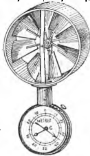
Fig. 125. Anemometru.
