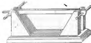
Fig. 4892. Termoscop.
