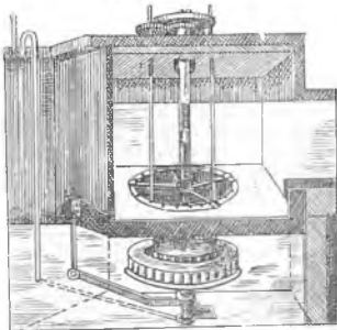
Fig. 5090. Turbină.
