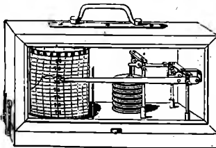
Fig. 386. Barometru inregistrator.
