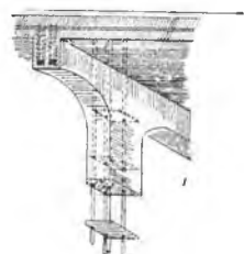
Fig. 458. Beton armat.
