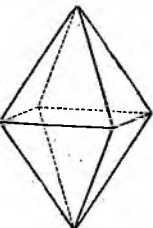
Fig. 4906. Piramidă tetragonală.
