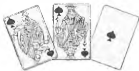
Fig. 4897. Terță majoră.
