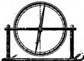
Fig. 176a. Declinațiune magnetică.
