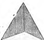
Fig. 4905. Tetraedru.
