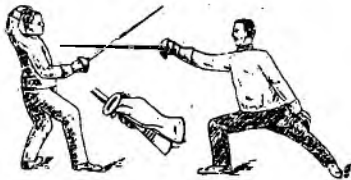
Fig. 4898. Terță.
