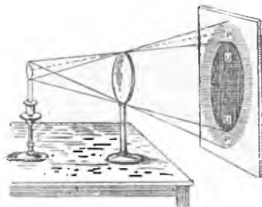
Fig. 3654. U.U. Umbra. - P.P. Penumbra.
