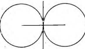
Fig. 4828. Tangentă.
