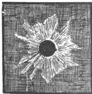
Fig. 1952. Eclipsă totală de soare.
