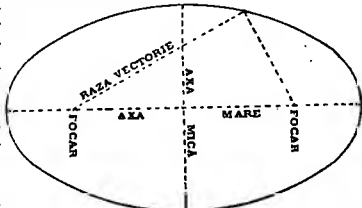
Fig. 1977. Elipsă.
