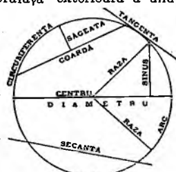
Fig. 1213. Circumferență.
