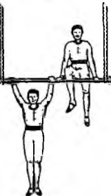
Fig. 5002. Trapez.
