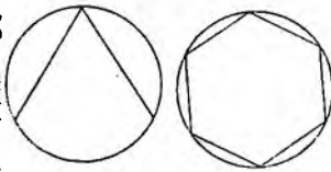
Fig. 2712. Unghi înșris. Fig. 2713. Poligon înșris.
