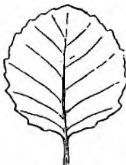
Fig. 1211. Frunză circulară.
