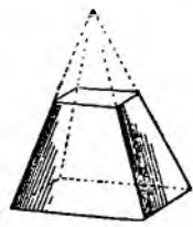
Fig. 5069. Trunchiul de piramidă.
