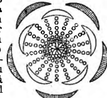
Fig. 1804. Diagrama trandafirului.
