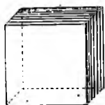
PARAL. CUB
