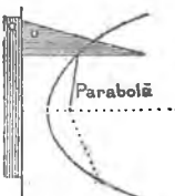
Fig. 3564. Parabolă.
