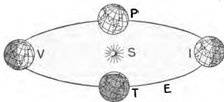
Fig. 1954. Ecliptica și pozițiunea pământului la diferitele anotimpuri.
