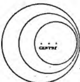
Fig. 2015. Cercuri excentrice.
