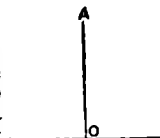
Fig. 3671. AO. Linie perpendiculară.
