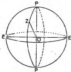
Fig. 3129. Meridianul ceresc. P. P. Linia polilor sferei cerești. EE. Ecuatorul ceresc. PZP. Meridianul ceresc al locului.
