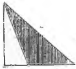
Fig. 4324. Triunghiur scalen.
