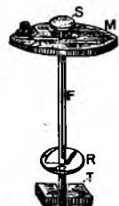
Fig. 4177. Roata olarului. S. Străgălic. — M. Masa. — F. Fusul. — R. Ro-tiță. — T. Tigaie.
