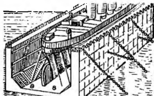
Fig. 1858. Dock plutitor.
