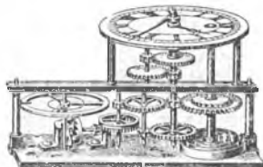
Fig. 3112. Mecanismul unui ceasornic de buzunar.
