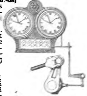
Fig. 2392. Girometru.
