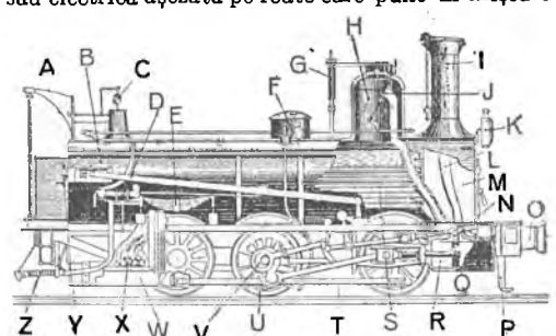
Fig. 2941. Locomotivă. A. Marchiza. — B. Cazan. — C. Fluier. — D. Injector de apă. — E. Resort. — F. Nisipar. — G. Balanță (supapă de siguranță). — H. Dom. — I. Coș. — J. Regulator. — K. Felinar. L. Teava de emisiune. — M. Cutia de fum. — N. Săltarul de distribuție. — O. Tampon. — P. Scară. — Q. Piston. — R. Cilindru. — S. Tevi de fum. — T. Biela. — U. Roată. — V. Excentric. — W. Cenușar. — X. Focar. — Y. Schimbătorul de mers. — Z. Teava de cuplare.
