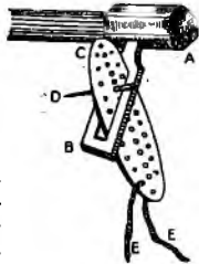
Fig. 106. Amnar (la războiu): A. Capătul sulului. - B. Amnar. - C. Lopățica. - D. Cuiu. - E. Sfoara ce leagă lopățica de patul războiului.
