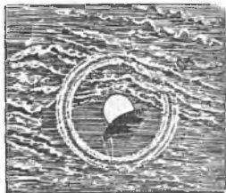
Fig. 1951. Eclipsă parțială de soare.
