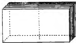
PARAL. DREPTUNGIULAR
