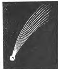
Fig. 1400. Cometă.
