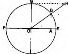
Fig. 1510. Cosecantă.
