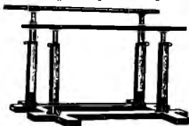
Fig. 3571. Paralele.
