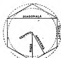
Fig. 3860. Poligon.
