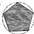
Fig. 3653. Pentagon.
