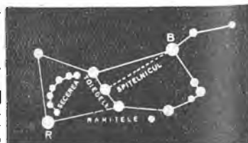
Fig. 4086. Rărițele (R. Rigel, - B. Betelgeuse).
