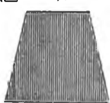
Fig. 5001. Trapez.
