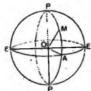
Fig. 176r. Declinațiunea unei stele.
