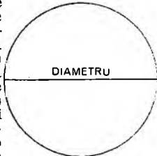
Fig. 1807. Diametru.
