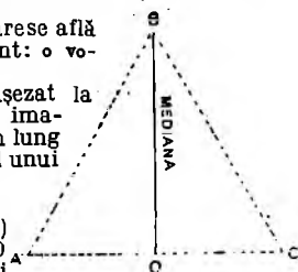
Fig. 3114. Mediană.
