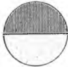
Fig. 4408. Semicerc.
