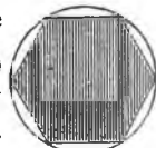
Fig. 2013. Exagon.
