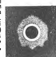
Fig. 2654. Eclipsă a inelară.
