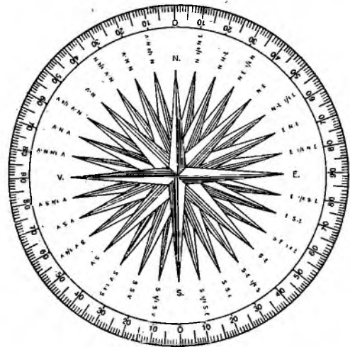
Fig. 4221. Roza vînturilor.
