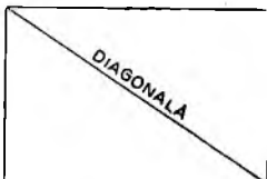
Fig. 1803. Diagonală.
