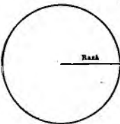
Fig. 4102. Rază.
