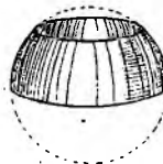
INEL SFERIC
