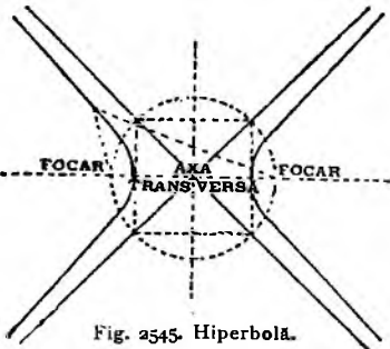
Fig. 2545. Hiperbolă.
