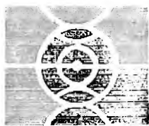
Fig. 2504. Halo.
