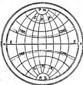
Fig. 3854. Poli. P.N. Polul nord. - P.S. Polul sud. - C.P.A. Cercul polar arctic. - C.P.A'. Cercul polar antarctic. - TRP. CNC. Tropicul Cancerului. - TRP. CPR. Tropicul Capricornului. - E. Ecuatorul.
