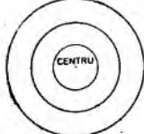
Fig. 1415. Cercuri concentrice.
