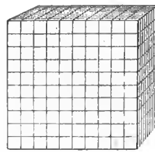
Fig. 1760. Decimetru cub împărțit în centimetri cubi (laturile reduse la 1/10).
