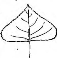
Fig. 1779. Frunză deltoidă.
