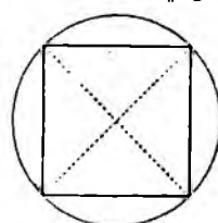
Fig. 1214. Cerc circumscriș.
