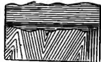
Fig. 1849. Straturi discordante.
