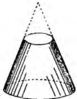
Fig. 5071. Trunchiul de con.
