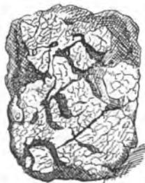
Fig. 33. Aerolit.
