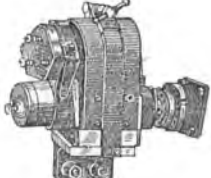
Fig. 3008. Magneto.
