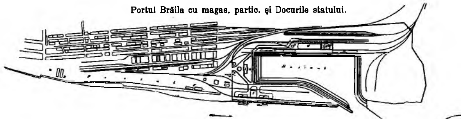
A. Serv. admin. și vamale, căpit. portului. B. Biroul magas. de cereale. C. Magas. „C. F. R.“ D. Debarcaderul vap. Reg. Stat. E. Usina electr. a serv. hidraulic. F. Pescărie. G. Magas. de cereale. I. Magas. p. mărf. întreprinsitate. M. Casa mașinelor. P. Platforme p. mărf. la aer liber. T. Mărf. transite.
