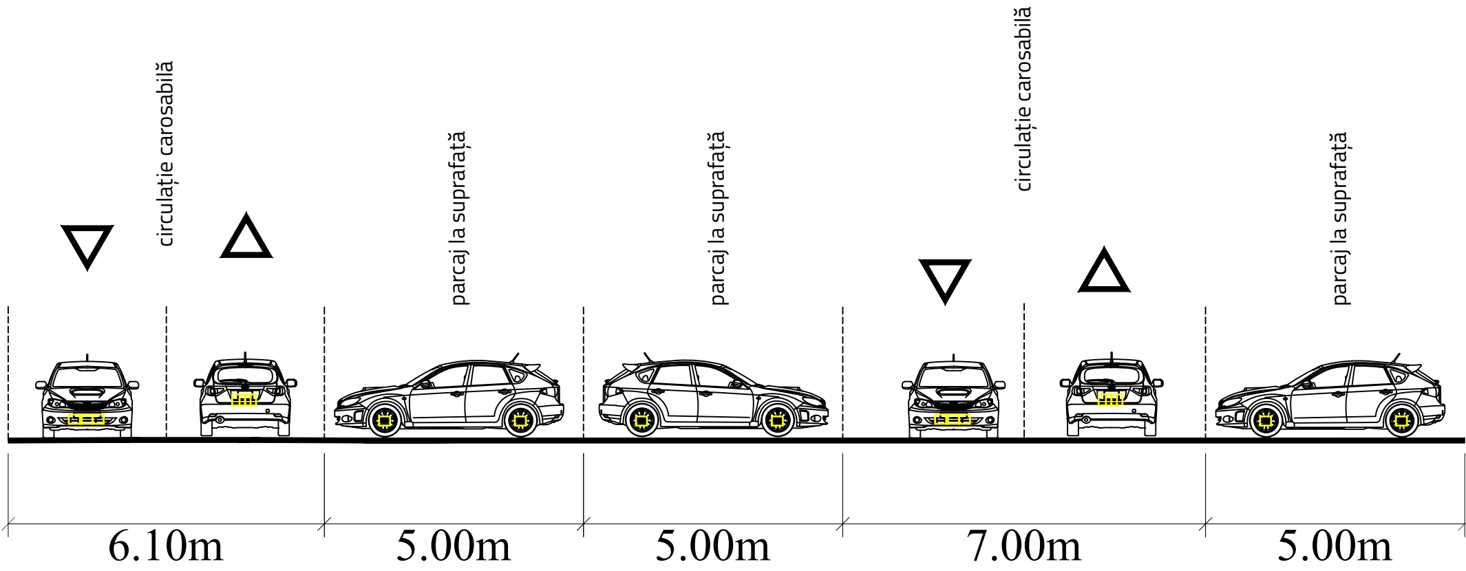
Drum incintă secțiune D-D1
