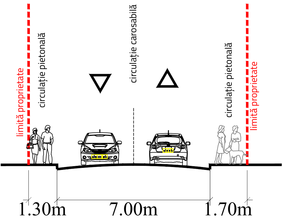
Sețiune 1-1a - Profil propus cf.HCL 172/2013;HCL nr. 258/2017.
