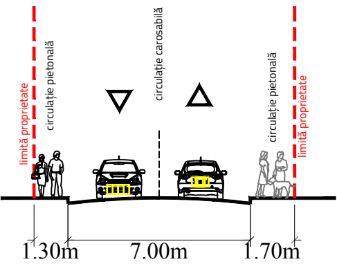
Secțiune AA' - Profil propus cf. HCL nr. 268/2013
