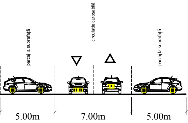
Drum incintă secțiune BB'
