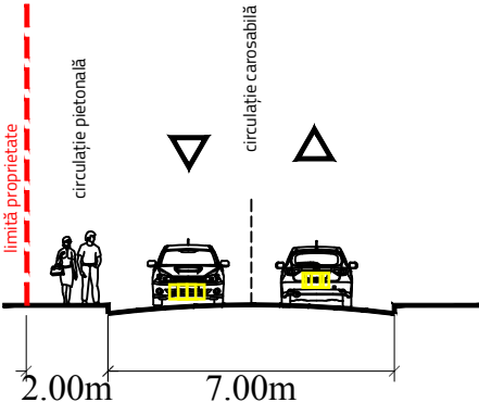
Drum incintă secțiune CC'
