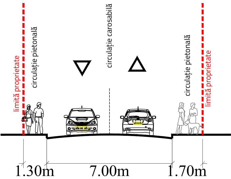
Secțiune 1-1a - Profil propus cf.HCL 172/2013, HCL nr. 258/2017
