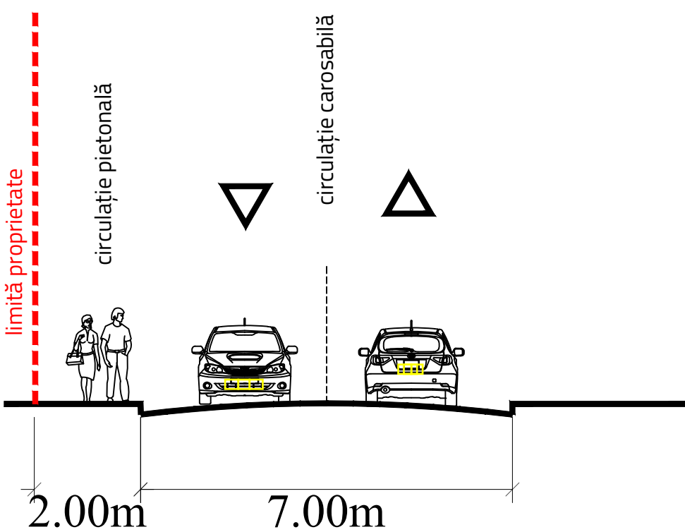
Drum incintă secțiune E-E1
