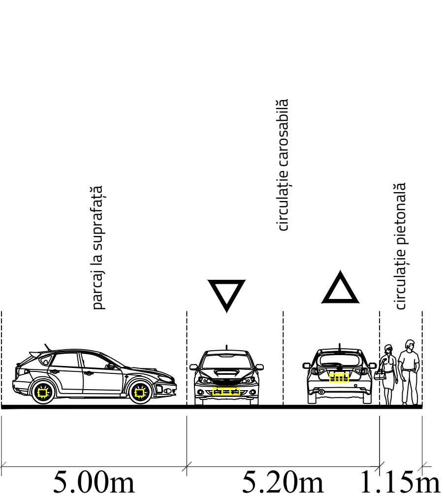
Drum incintă secțiune C-C1
