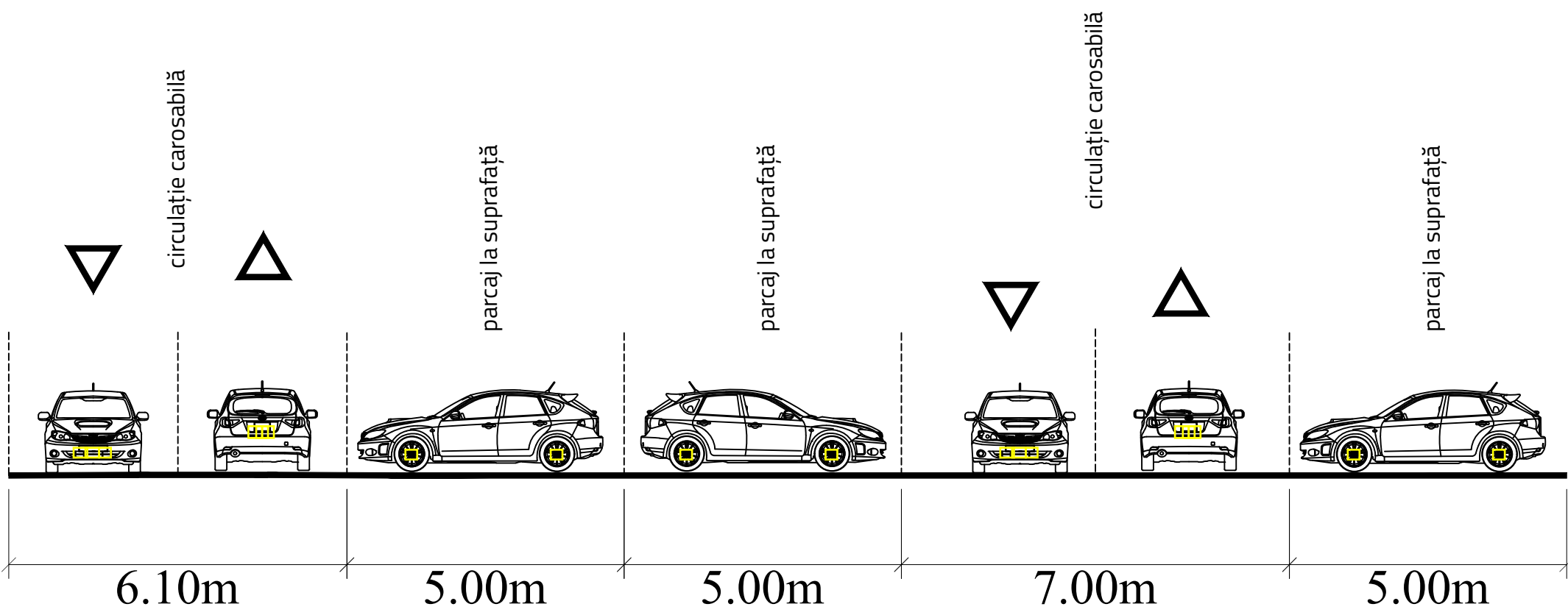
Drum incintă secțiune D-D1
