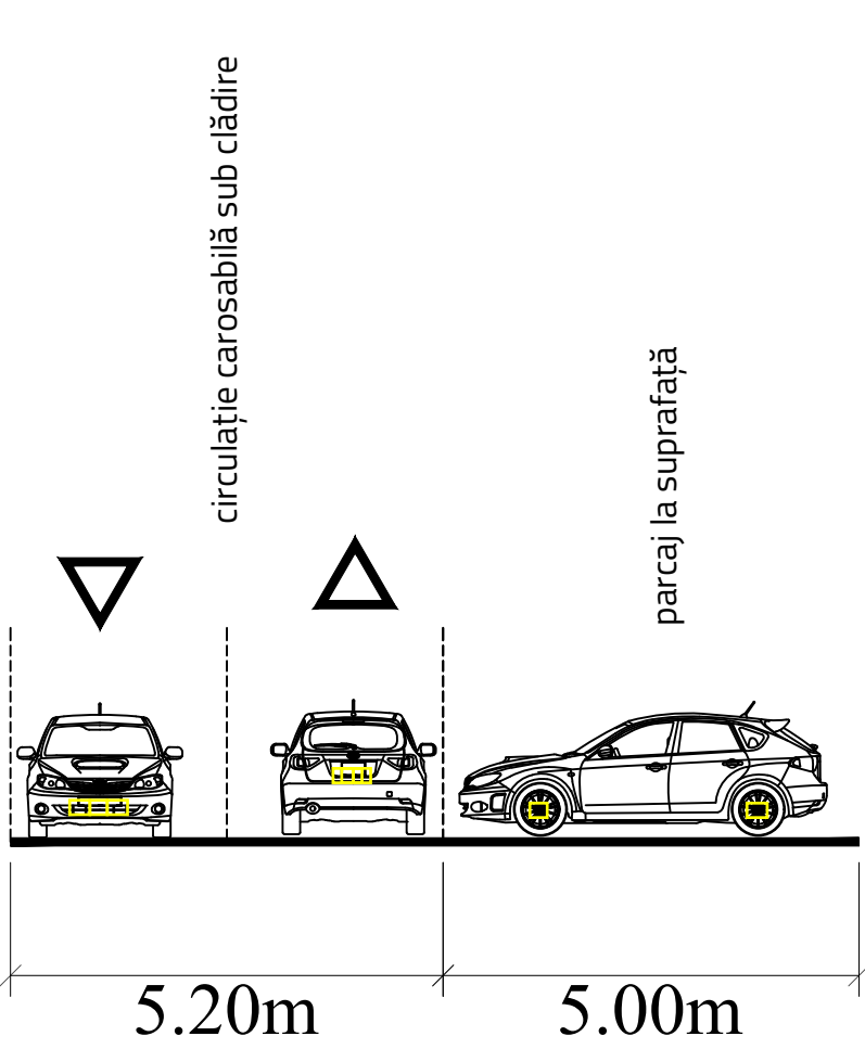
Drum incintă secțiune B-B1
