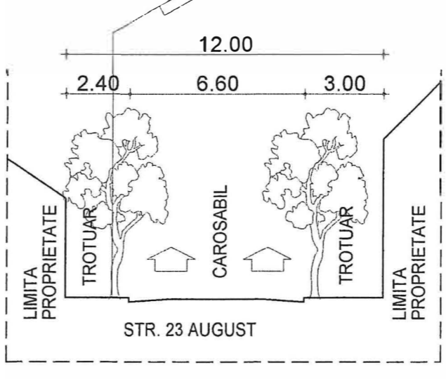
PROFIL STRADAL PS1
