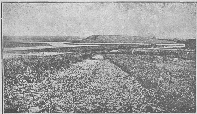
Stânca Bisericuța și gârla Ciulinețul.
