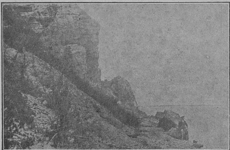
Ţărml cretacic al lacului Razim (Capul Dolojman)
