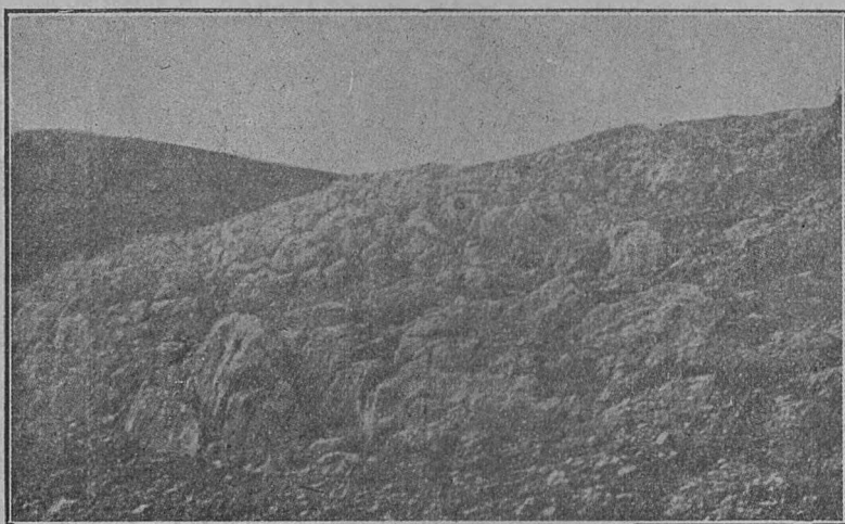
Calcarurile triasice dela Enisala.
