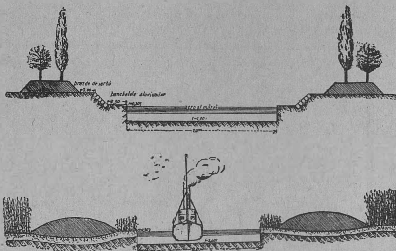
(C) secțiune în regiunea plaurului din Delta Dunării (după dr. Antipa)
