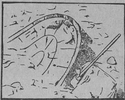
Un anticlinal în calcarurile triasice din Niculițel-Tulcea. (După o fotografie luată de M. Savul).
