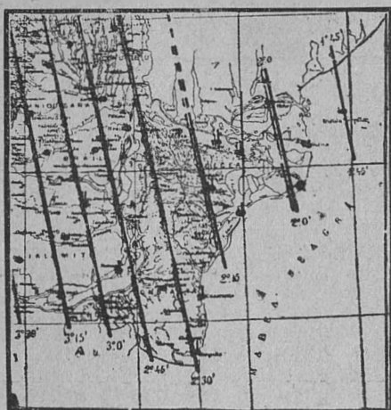
Declinația magnetică la 1 Ianuarie 1906. Componenta orizontală a puterii magnetice.
