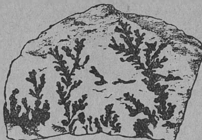
Dendrite pe granitul dela Măcin (Originalul se găsește la laboratorul geologic din Iași).
