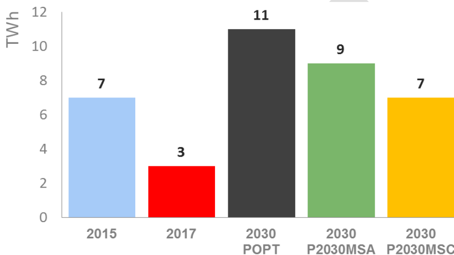
Figura 10 – Exportul net de energie electrică (Sursa: PRIMES)
