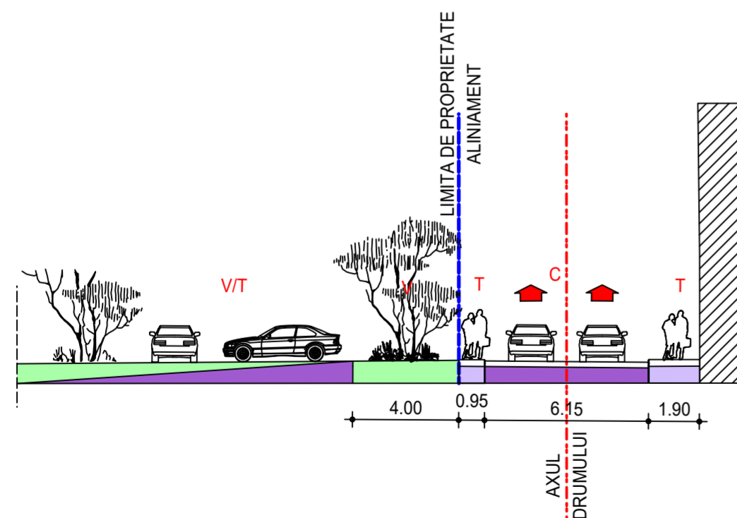
SECTIUNE - PROFIL 5:5 - STR. ION ROATA
