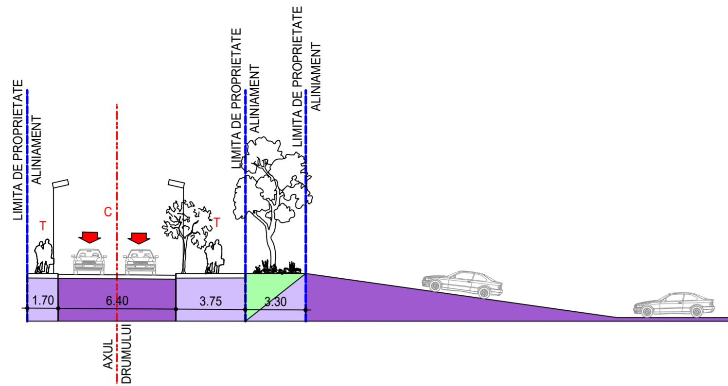
SECTIUNE - PROFIL 1:1 - STR. DUMITRU MARINESCU
