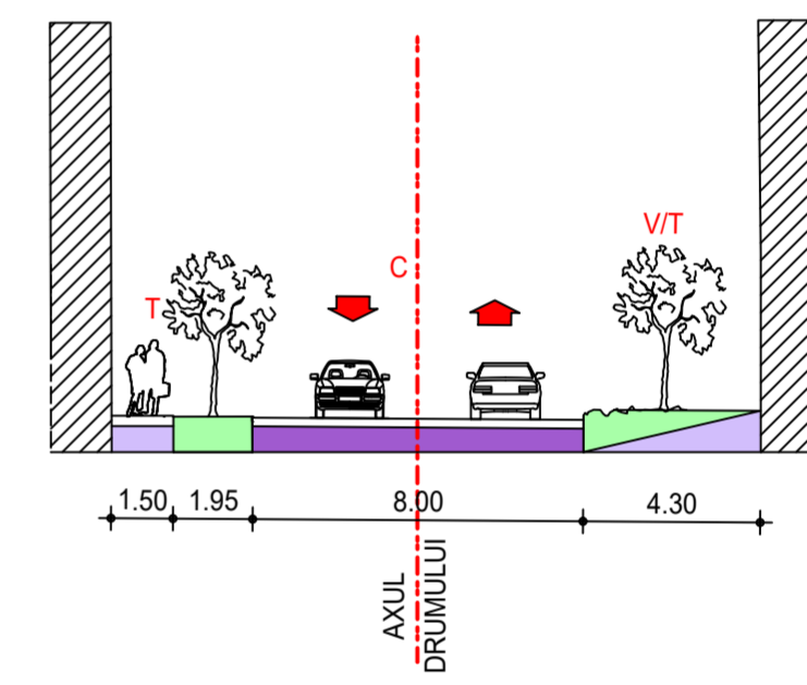
SECTIUNE - PROFIL 4:4 - STR. STRADA INTERIOARA 1
