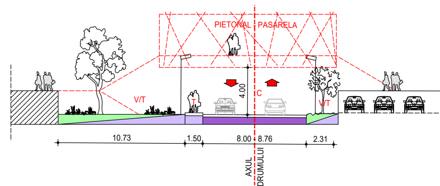
SECTIUNE - PROFIL 6:6 - STR. INTERIOARA 1
