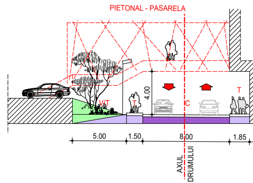
SECTIUNE - PROFIL 3:3 - STRADA INTERIOARA 1
