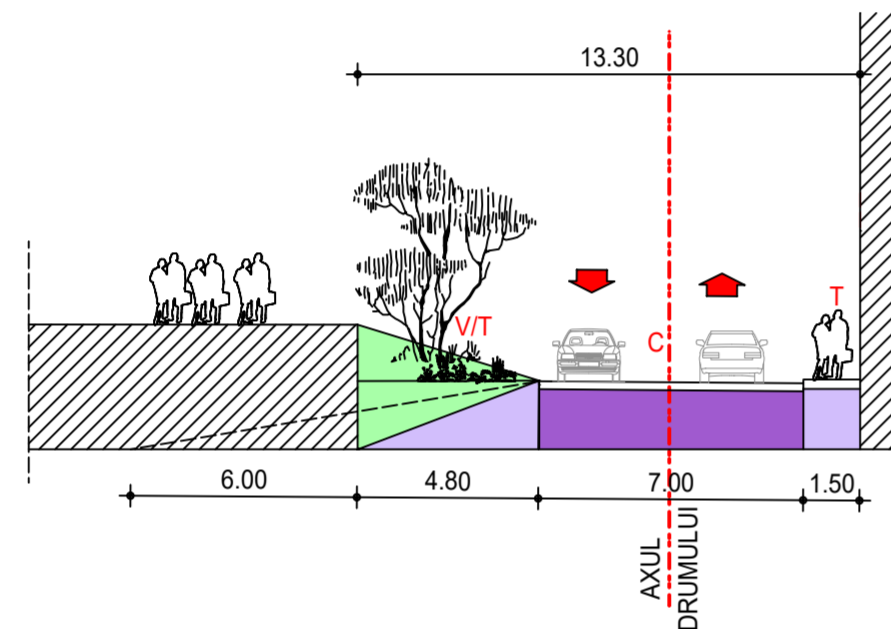
SECTIUNE - PROFIL 2:2 - STRADA INTERIOARA 2
