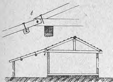
Secțiunea transversală a casei.
