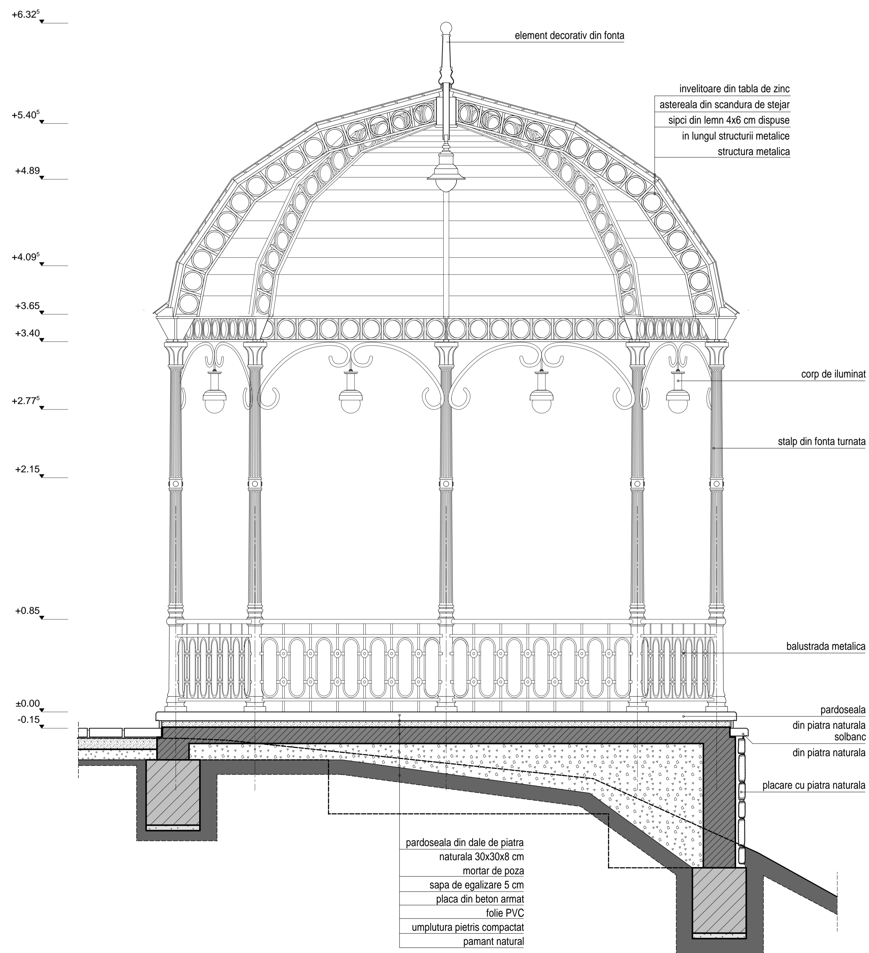
SECTIUNE TRANSVERSALA DIAGONALA
